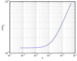
FIG. 6.25. err_p
