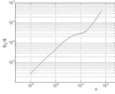
FIG. 6.8. err(u)
