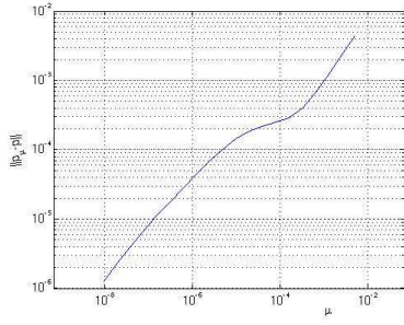
FIG. 6.10. err(p)
