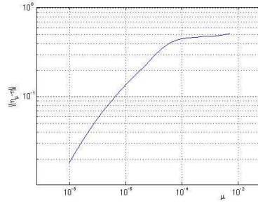
FIG. 6.11. err(\eta)
