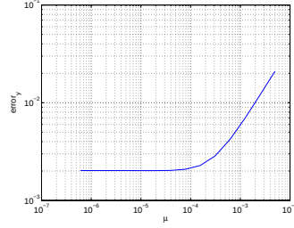
FIG. 6.24. err_y
