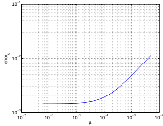
FIG. 6.23. err_u
