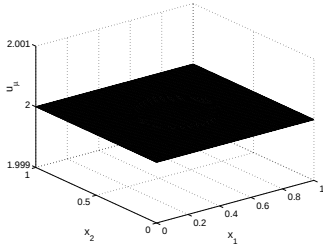
FIG. 6.4. Control u_h
