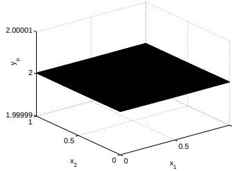
FIG. 6.5. State y_h
