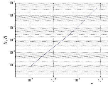
FIG. 6.9. err(y)
